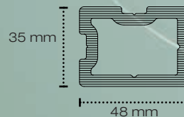
P 9554/P 9544
